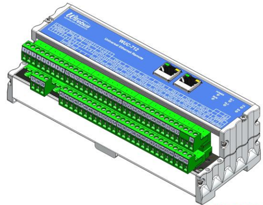
VISTA ISOMÉTRICA
