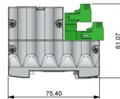
VISTA LATERAL
