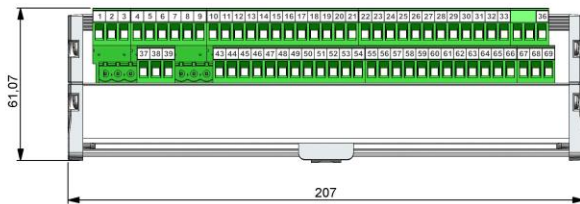
VISTA INFERIOR
