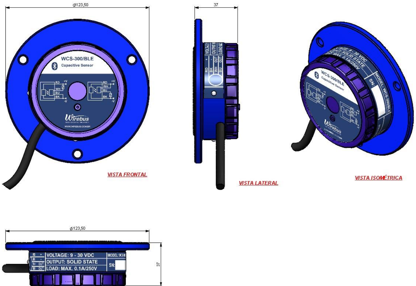
Figura 1. Dimensões.
